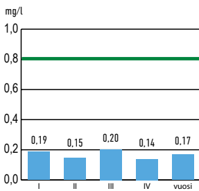
Käsitellyn jäteveden fosforipitoisuus 2025 Luparaja 0,8 mg/l
