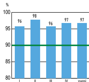
Kiintoaineen puhdistusteho 2025 Luparaja 90 %
