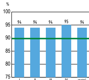
COD c :n puhdistusteho 2025 Luparaja 90 %
