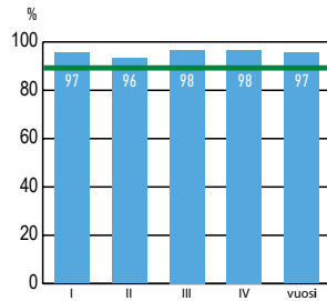
BOD 7 :n puhdistusteho 2025 Luparaja 92 %
