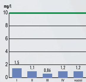
Käsitellyn jäteveden BOD 7 ATU-pitoisuus 2025 Luparaja 10 mg/l
