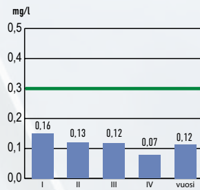
Käsitellyn jäteveden fosforipitoisuus 2025 Luparaja 0,3 mg/l
