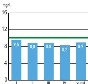
Käsitellyn jäteveden kiintoainepitoisuus 2025 Luparaja 10 mg/l
