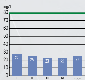
Käsitellyn jäteveden CODCr-pitoisuus 2025 Luparaja 80 mg/l
