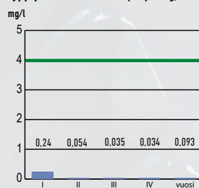
Käsitellyn jäteveden ammoniumtyppipitoisuus 2025 Luparaja 4 mg/l
