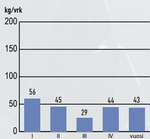
Käsitellyn jäteveden BOD 7 ATU:n kuormitus vesistöön 2025
