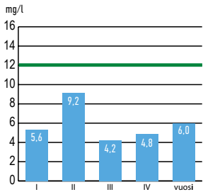
Käsitellyn jäteveden BOD 7 -pitoisuus 2025 Luparaja 12 mg/l
